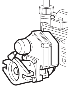
Flangiatura con riduttore e disinnesto Flange with red. gear and disconnect Brida con reductora y desembrage Bride avec réducteur et débrayage Flansch mit Untersetzungsgetriebe und Ausrückvorrichtung
