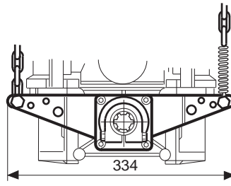
Attacco rapido 1"3/8 F. Quick coupler 1"3/8 F. Enganche 3 puntos toma de fuerza H. 1"3/8 Prise rapide 1"3/8 F. 3-Punkt Schnellschluß 1"3/8 mit Ketten
